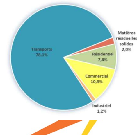
ÉMISSIONS DE GES COLLECTIVITÉ PAR SECTEUR
