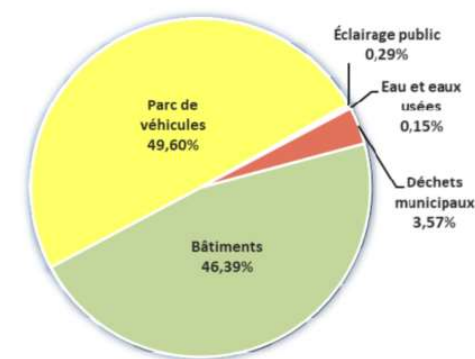
ÉMISSIONS DE GES COLLECTIVITÉ PAR SECTEUR
